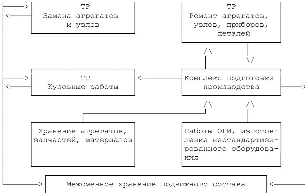
Рис. 1. Схема технологического процесса ТО и ТР подвижного состава
