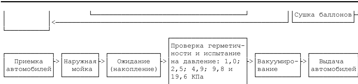
Рис. 3. Схема технологического процесса переосвидетельствования автомобильных баллонов для СПГ и СНГ и испытания топливных систем автомобилей, работающих на СПГ
