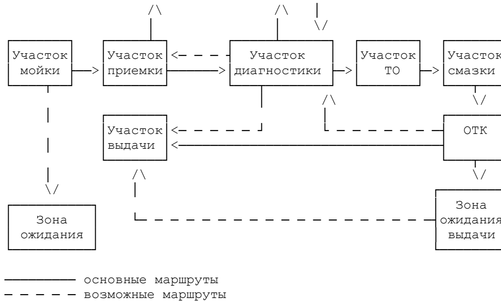
Рис. 4. Схема производственного процесса полнообъемного ТО на СТОА
