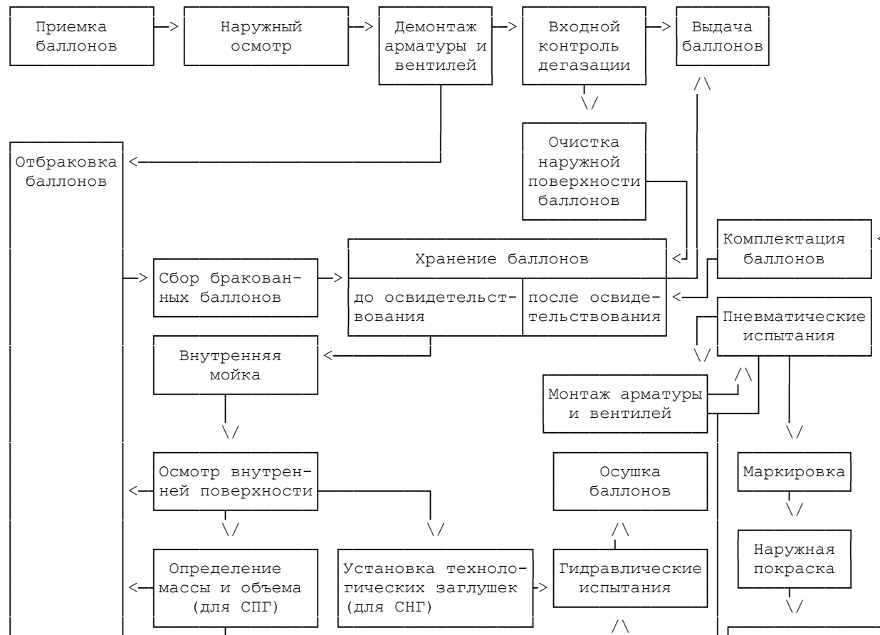
Рис. 2. Схема технологического процесса текущего ремонта агрегатов и узлов на ЦСП
