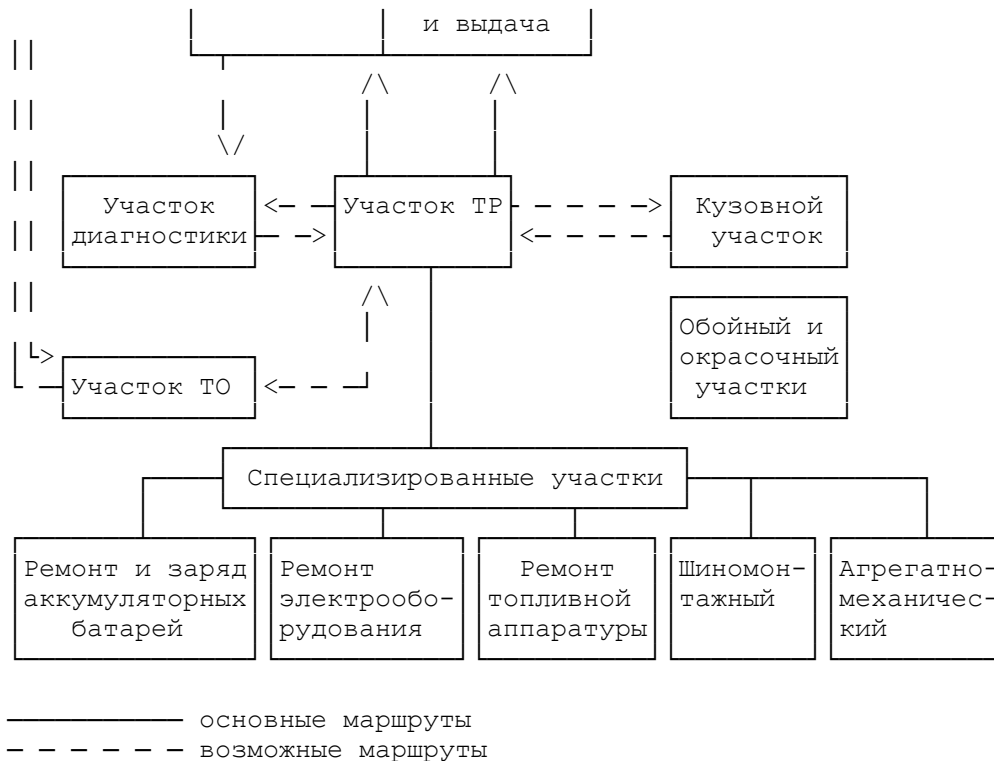
Рис. 5. Схема технологического процесса ТР на СТОА
